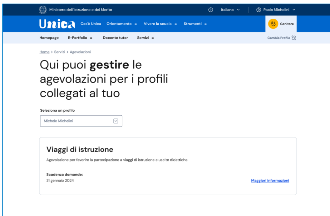
FIGURA 25 – SCHERMATA AGEVOLAZIONI
